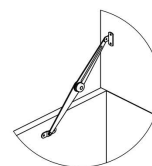
左限位器安装示意图
