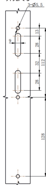
开孔尺寸
