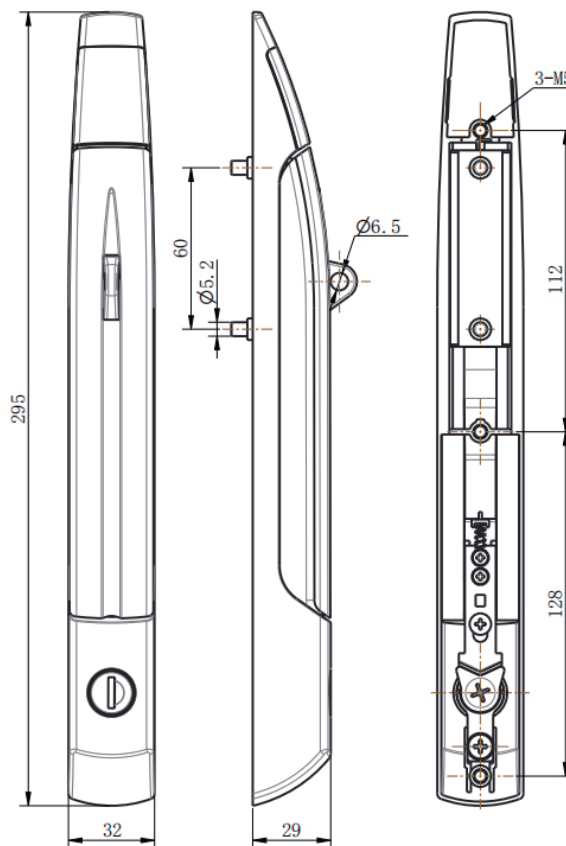
开孔尺寸
